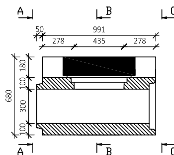
BEST ČISTIČÍ KUS ZÁKLADNÍ 20/30 (PERO-DŘÁŽKA), OBRUBNÍK 18 cm (PROFIL LEVÝ)
