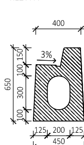
ŘEZ A-A
