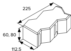
BEST BASE kraj
