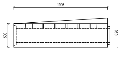
POHLED A-A
