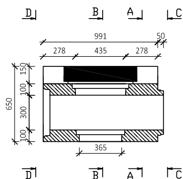
BEST VPUSŤOVÝ KUS 20/30 (PERO-DŘÁŽKA), OBRUBNÍK 15 cm (PROFIL PRAVÝ)
