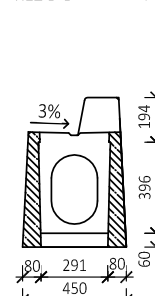
ŘEZ B-B
