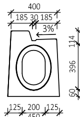
BEST ČISTIČÍ KUS VRCHOLOVÝ 20/20 (PERO-PERO), OBRUBNÍK 7 cm (PROFIL PRAVÝ/LEVÝ)
