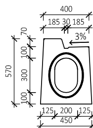
BEST VPUŠŤOVÝ KUS 20/30 (PERO-DŘÁŽKA), OBRUBNÍK 7 cm (PROFIL LEVÝ)
