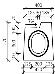
BEST VPUŠŤOVÝ KUS 20/30 (PERO-DŘÁŽKA), OBRUBNÍK 7 cm (PROFIL PRAVÝ)
