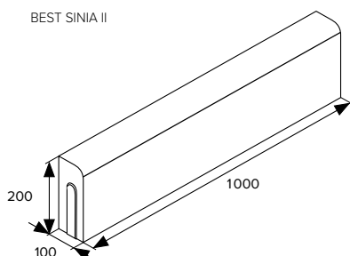
BEST SINIA II
