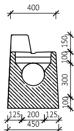
ŘEZ B-B
