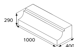
BEST ZASTÁVKOVÝ OBRUBNÍK přímý 290
