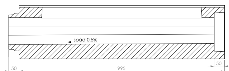
BEST MALÁ TROUBA S PRŮBĚŽNÝM ŠTĚRBINOVÝM ŽLABEM, SPÁDOVÉ JÁDRO 125/130
