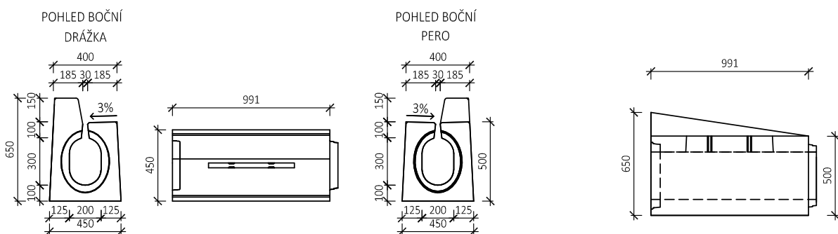
BEST TROUBA SE ŠTĚRBINOVÝM ŽLABEM, NÁBĚHOVÁ 0-15, OBRUBNÍK 15 cm (PROFIL PRAVÝ)
