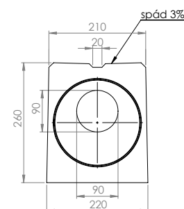
BEST MALÁ TROUBA S PRŮBĚŽNÝM ŠTĚRBINOVÝM ŽLABEM, SPÁDOVÉ JÁDRO 90/95
