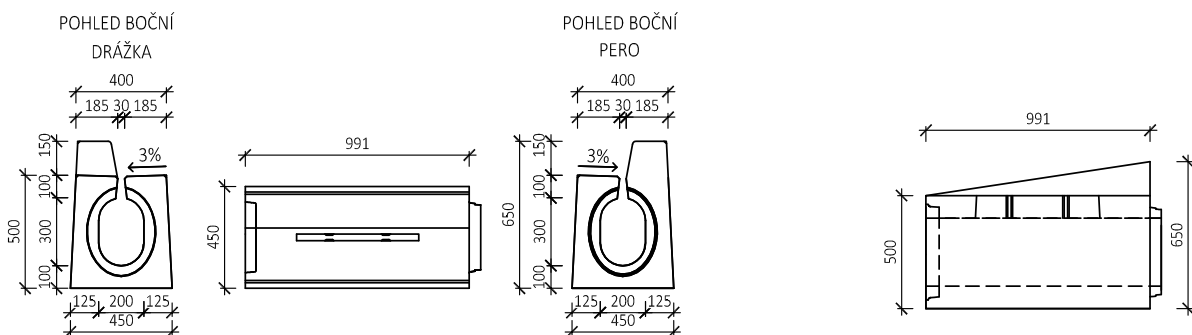
BEST TROUBA SE ŠTĚRBINOVÝM ŽLABEM, NÁBĚHOVÁ 15-0, OBRUBNÍK 15 cm (PROFIL PRAVÝ)
