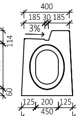
BEST VPUŠŤOVÝ KUS (DŘÁŽKA-DŘÁŽKA), OBRUBNÍK 7 cm (PROFIL PRAVÝ/LEVÝ)
