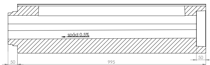
BEST MALÁ TROUBA S PRŮBĚŽNÝM ŠTĚRBINOVÝM ŽLABEM, SPÁDOVÉ JÁDRO 120/125
