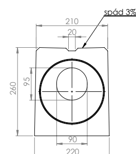
BEST MALÁ TROUBA S PRŮBĚŽNÝM ŠTĚRBINOVÝM ŽLABEM, SPÁDOVÉ JÁDRO 95/100
