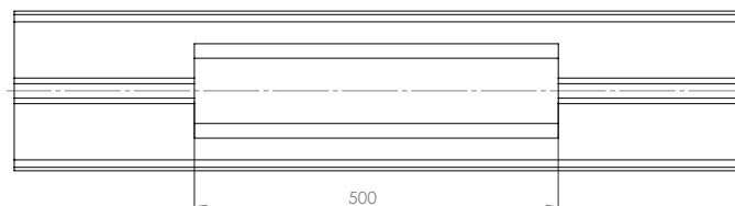
BEST MALÝ VPUŠŤOVÝ KUS ZÁKLADNÍ, ROVNÉ JÁDRO 140/140
