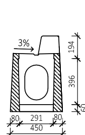
ŘEZ B-B
