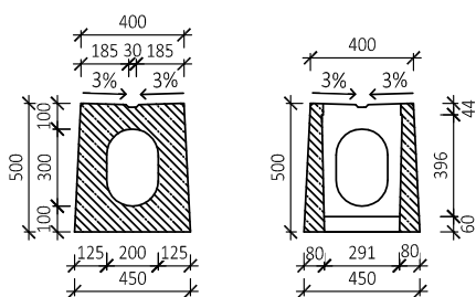
BEST ZÁSLEPKA TROUBY SE ŠTĚRBINOVÝM ŽLABEM ZAKONČENÁ DŘÁŽKOU
