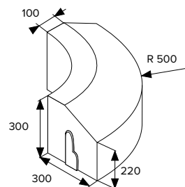
BEST RONDA R0,5 vnější
