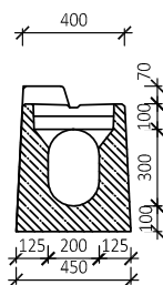
BEST VPUŠŤOVÝ KUS 20/30 (PERO-DŘÁŽKA), OBRUBNÍK 7 cm (PROFIL PRAVÝ)
