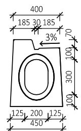
BEST VPUŠŤOVÝ KUS 20/30 (PERO-DŘÁŽKA), OBRUBNÍK 7 cm (PROFIL PRAVÝ)
