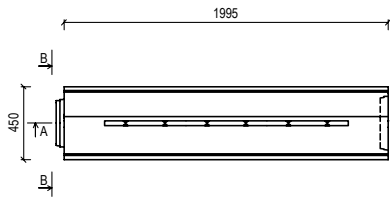
PŮDORYS
