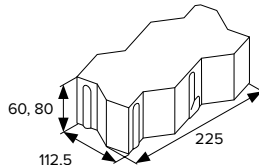
BEST BASE rovná
