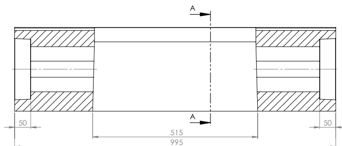
BEST MALÝ VPUŠŤOVÝ KUS ÚŽLABNÍ, ROVNÉ JÁDRO 140/140
