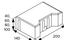
BEST BEATON kraj
