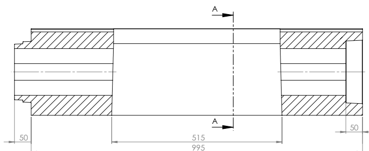
BEST MALÝ VPUŠŤOVÝ KUS ZÁKLADNÍ, ROVNÉ JÁDRO 140/140
