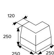
BEST MONO II rohový 90 vnější
