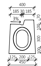
BEST VPUŠŤOVÝ KUS 20/30 (PERO-DŘÁŽKA), OBRUBNÍK 7 cm (PROFIL LEVÝ)
