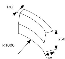
BEST MONO II R1 vnitřní
