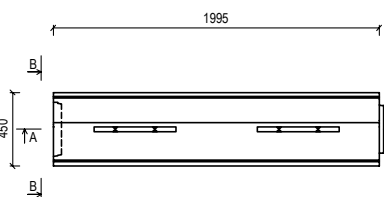
PŮDORYS
