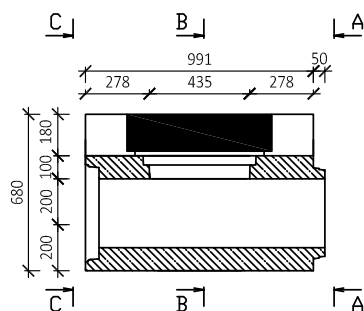
BEST ČISTIČÍ KUS ZÁKLADNÍ 20/30 (PERO-DŘÁŽKA), OBRUBNÍK 18 cm (PROFIL PRAVÝ)
