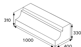
BEST ZASTÁVKOVÝ OBRUBNÍK náběhový 310/330
