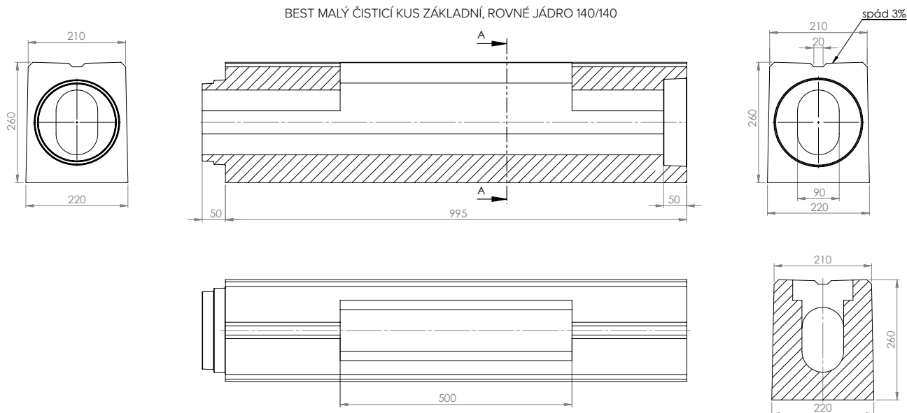
BEST MALÝ ČISTICÍ KUS ZÁKLADNÍ, ROVNÉ JÁDRO 140/140
