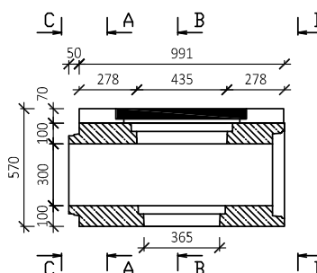
ŘEZ B-B
