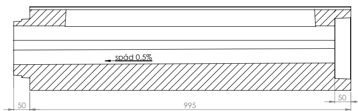
BEST MALÁ TROUBA S PRŮBĚŽNÝM ŠTĚRBINOVÝM ŽLABEM, SPÁDOVÉ JÁDRO 115/120
