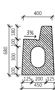
ŘEZ A-A
