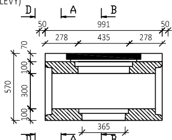
ŘEZ B-B
