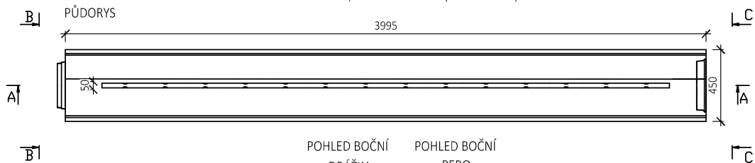
BEST TROUBA S PRŮBĚŽNÝM ŠTĚRBINOVÝM ŽLABEM, OBRUBNÍK 7 cm (PROFIL LEVÝ)
