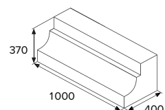
BEST ZASTÁVKOVÝ OBRUBNÍK přímý 370
