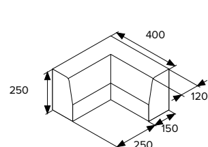
BEST MONO II rohový 90 vnitřní
