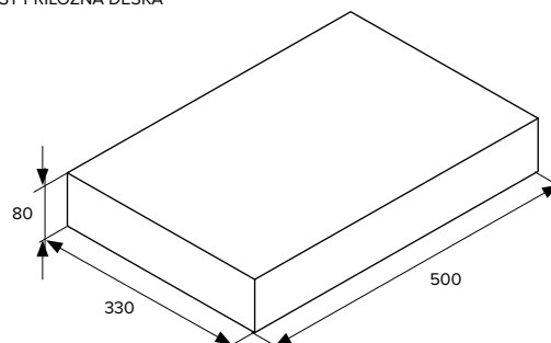
BEST PŘÍLOŽNÁ DESKA
