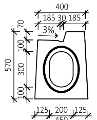
BEST ČISTIČÍ KUS VRCHOLOVÝ 20/20 (PERO-PERO), OBRUBNÍK 7 cm (PROFIL PRAVÝ/LEVÝ)
