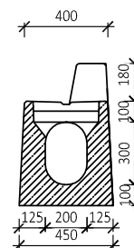
ŘEZ B-B
