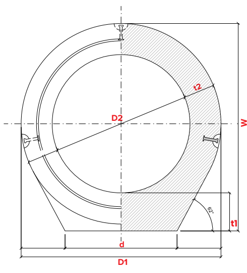
PŘÍČNÝ ŘEZ
