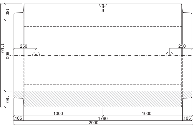
PATKOVÁ TROUBA TZP-SP 80/200 DD
