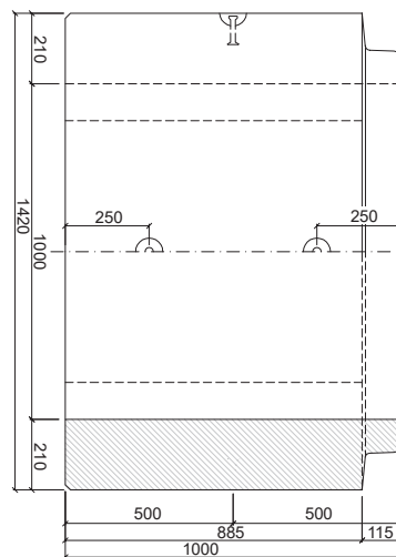
PATKOVÁ TROUBA TZP-SP 100/100 KD
