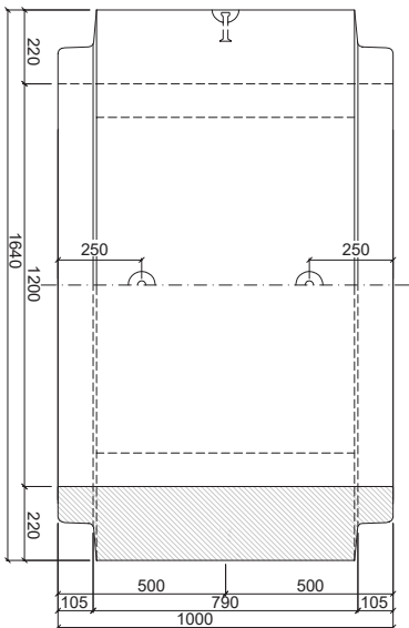
PATKOVÁ TROUBA TZP-ZP 120/100 DD
