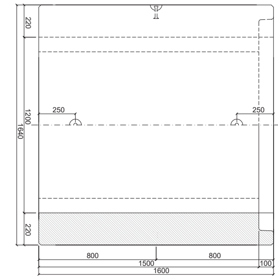
PATKOVÁ TROUBA TZP-ZP 120/150 KH
