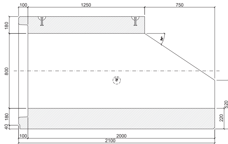
PATKOVÁ TROUBA TZP-ZP 80/200/125 SH
