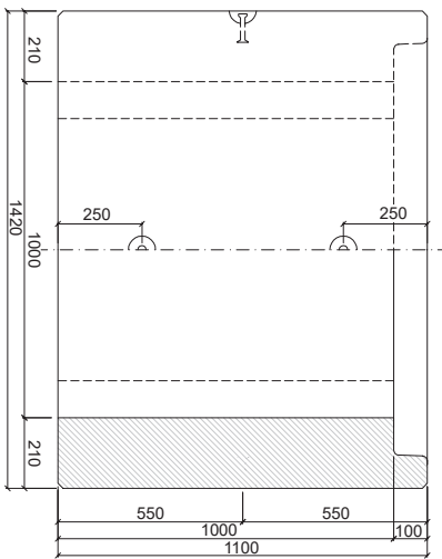
PATKOVÁ TROUBA TZP-ZP 100/200 KH
