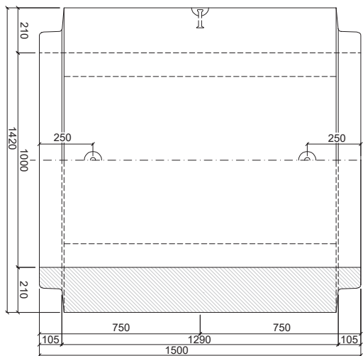
PATKOVÁ TROUBA TZP-SP 100/150 DD
