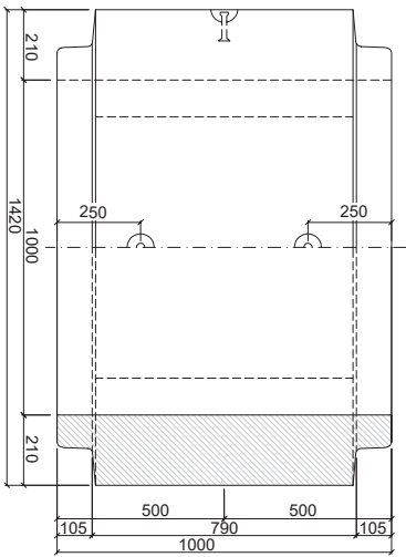
PATKOVÁ TROUBA TZP-ZP 100/100 DD
