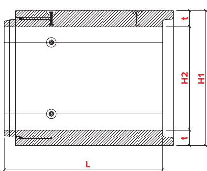
PODÉLNÝ ŘEZ
