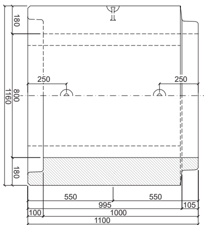
PATKOVÁ TROUBA TZP-SP 80/100 HD
