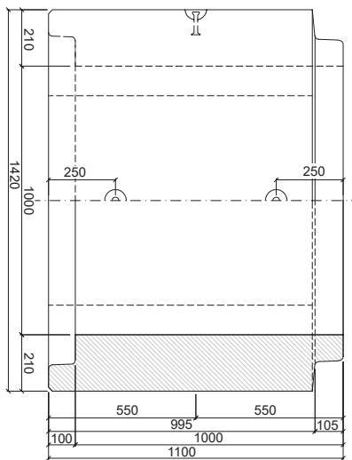
PATKOVÁ TROUBA TZP-SP 100/200 HD
