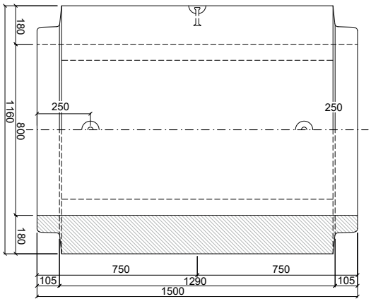
PATKOVÁ TROUBA TZP-ZP 80/150 DD
