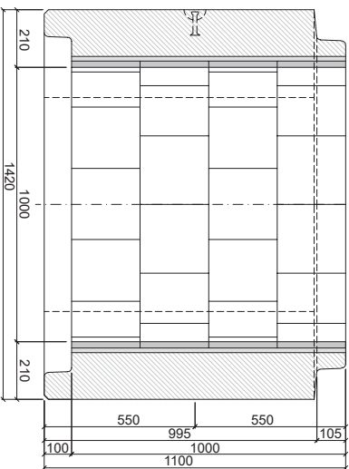
PATKOVÁ TROUBA TZP-SP 100/200 HDOC
