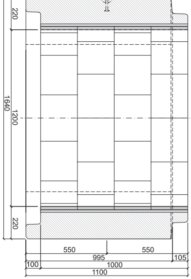
PATKOVÁ TROUBA TZP-SP 120/200 HDOC
