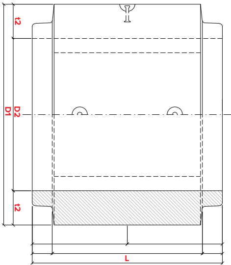
POHLED ZE SHORA / PODÉLNÝ ŘEZ
