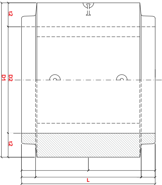
POHLED ZE SHORA / PODÉLNÝ ŘEZ
