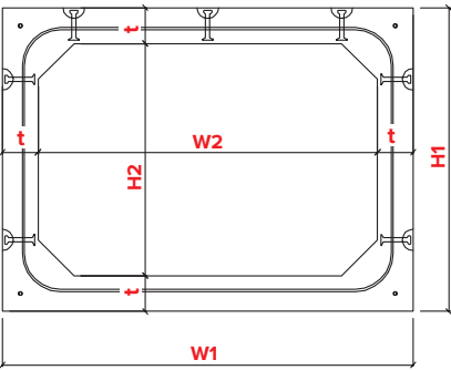
PŘÍČNÝ ŘEZ
