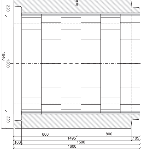
PATKOVÁ TROUBA TZP-SP 120/150 HDOC
