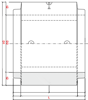
POHLED ZE SHORA / PODÉLNÝ ŘEZ
