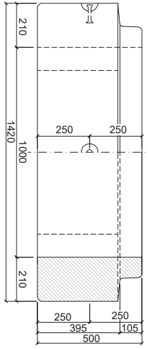
PATKOVÁ TROUBA TZP-ZP 100/50 KD
