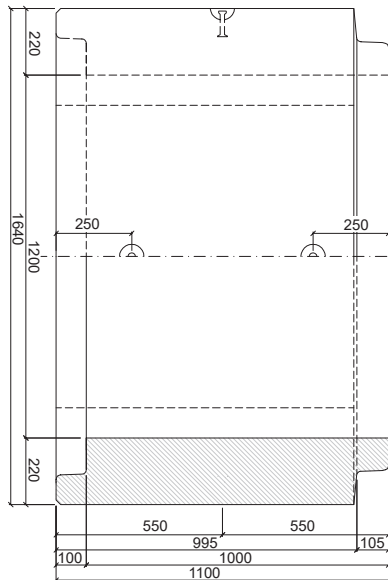
PATKOVÁ TROUBA TZP-SP 120/100 HD
