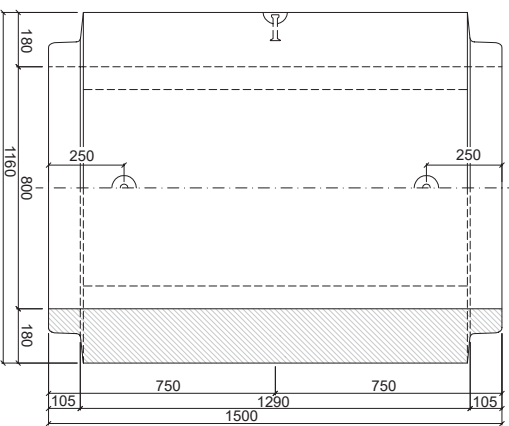
PATKOVÁ TROUBA TZP-SP 80/150 DD
