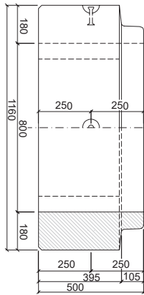
PATKOVÁ TROUBA TZP-ZP 80/50 KD
