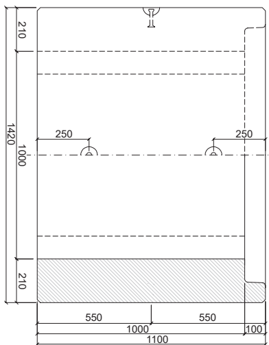
PATKOVÁ TROUBA TZP-SP 100/100 KH
