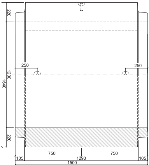
PATKOVÁ TROUBA TZP-ZP 120/150 DD
