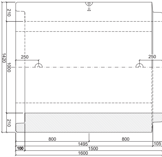
PATKOVÁ TROUBA TZP-ZP 100/150 HD
