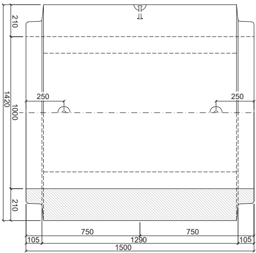
PATKOVÁ TROUBA TZP-ZP 100/150 DD
