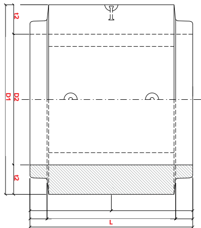
POHLED ZE SHORA / PODÉLNÝ ŘEZ
