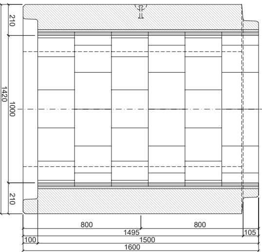
PATKOVÁ TROUBA TZP-SP 100/150 HDOC
