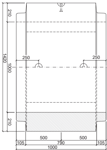
PATKOVÁ TROUBA TZP-SP 100/100 DD
