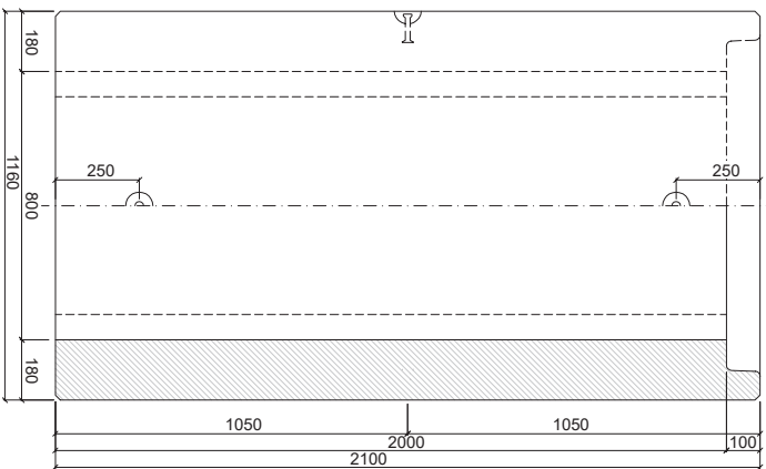
PATKOVÁ TROUBA TZP-ZP 80/200 KH
