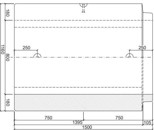
PATKOVÁ TROUBA TZP-SP 80/100 KD
