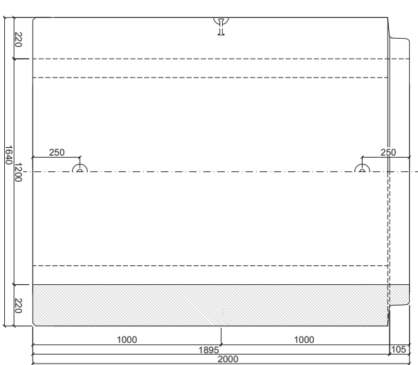
PATKOVÁ TROUBA TZP-ZP 120/200 KD
