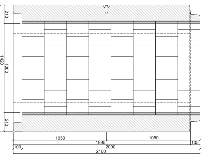
PATKOVÁ TROUBA TZP-SP 100/200 HDOC
