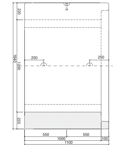
PATKOVÁ TROUBA TZP-ZP 120/100 KH
