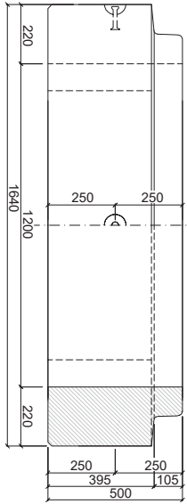
PATKOVÁ TROUBA TZP-ZP 120/50 KD
