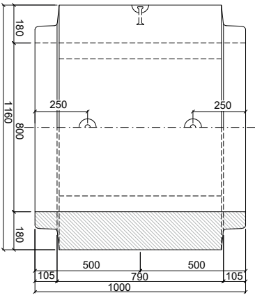
PATKOVÁ TROUBA TZP-ZP 80/100 DD
