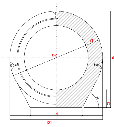
POHLED ČELNÍ / PŘÍČNÝ ŘEZ
