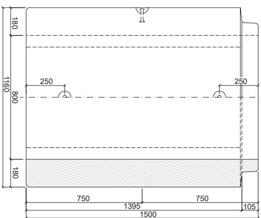
PATKOVÁ TROUBA TZP-SP 80/150 KD
